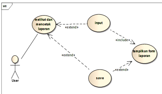
Gambar 4 Use Case Diagram Mencetak Laporan
