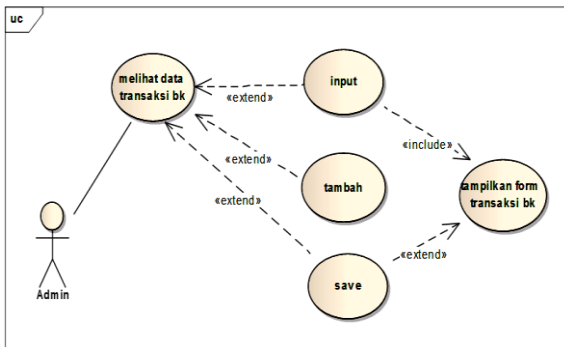
Gambar 3 Use Case Diagram Mengelola Data Transaksi Barang Masuk
