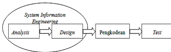
Gambar 1 Tahapan-Tahapan SDLC
