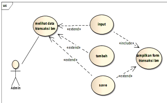
Gambar 2 Use Case Diagram Mengelola Data Transaksi Barang Masuk
