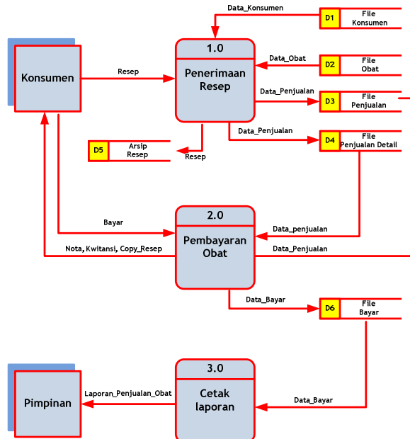
Gambar 2 Diagram Nol Sistem Penjualan Obat
