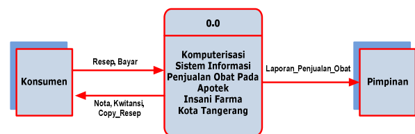
Gambar 1 Diagram Konteks Sistem Informasi Penjualan Obat
